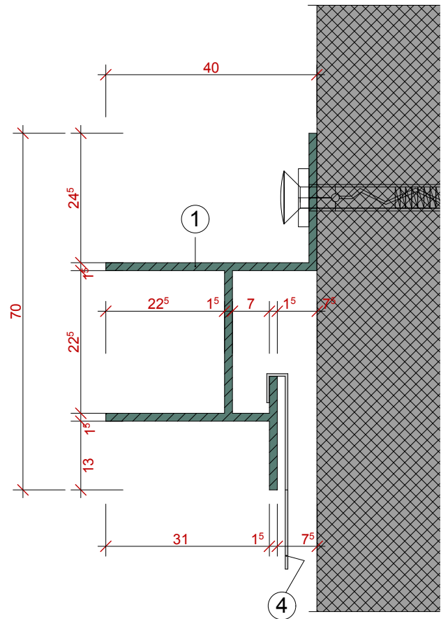
Querschnitt Galeria - Profil Msst. 1:1
